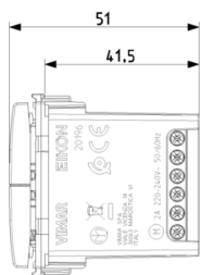
Vista ingombri
