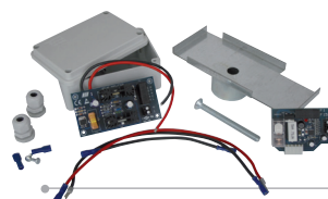
AD00318 SET SOLAR AMPLIFIER per K800 24V. Amplificatore di voltaggio per 2 pannelli solari fino a 200W 12V cadauno
