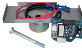
ACG4662 CARICA BATTERIA per K800 24V con supporto per le batterie da 2,2Ah (ACG9515 x 2)
