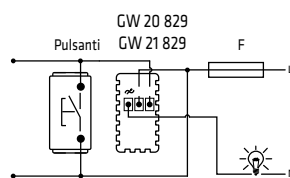
Comando e regolazione da due punti (1 dimmer + 1 pulsante NA)
