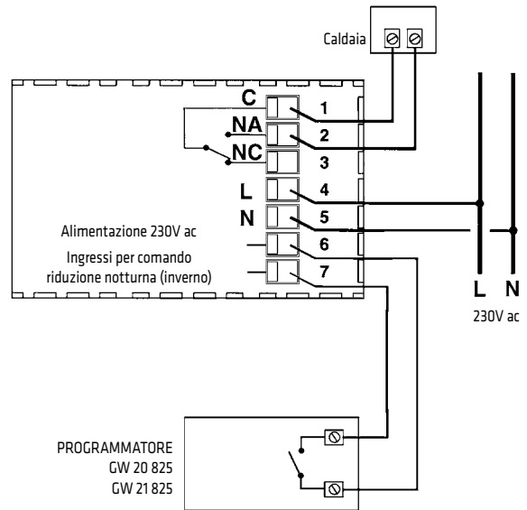
Esempio di collegamento a caldaia e orologio per comando riduzione notturna
