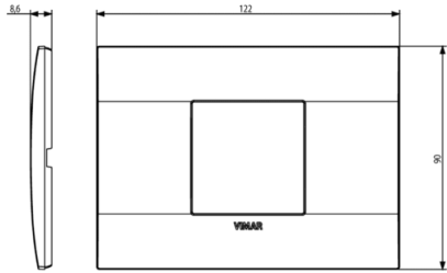
Vista ingombri
