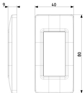
Vista ingombri
