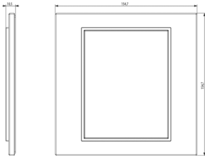
Vista ingombri
