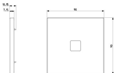
Vista ingombri
