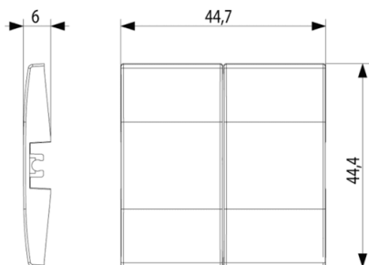
Vista ingombri
