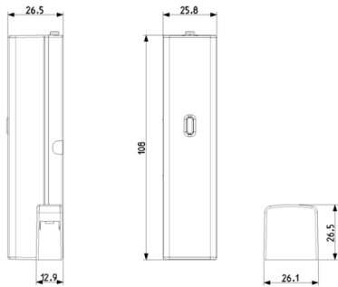
Vista ingombri
