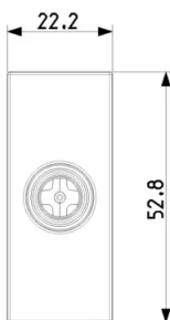
Vista ingombri
