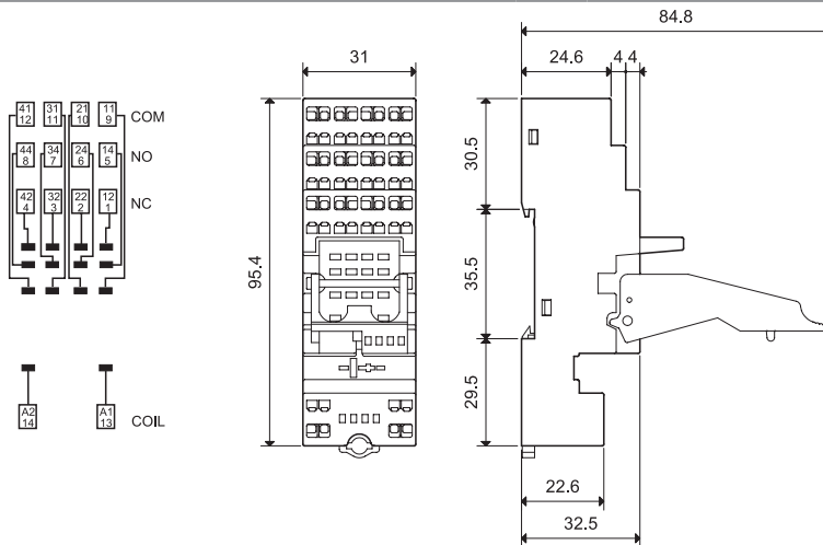
Zoccolo + Pettine
