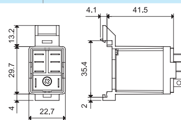
056.27 con relè
