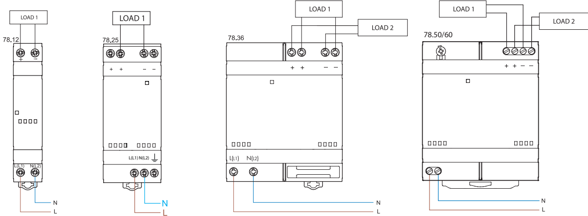
Collegamento a doppia polarità
