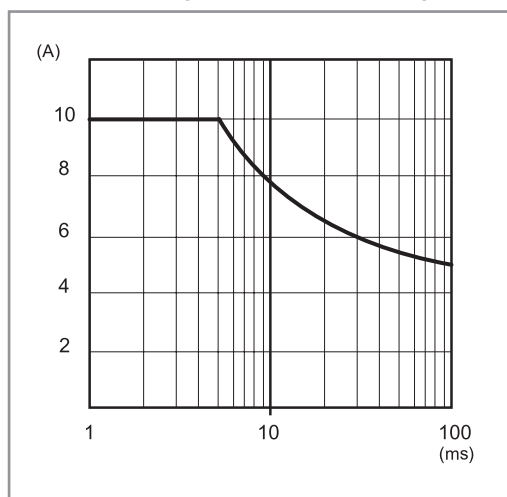
P78-9 Corrente di picco in funzione del tempo (78.1D)
