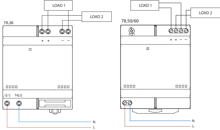
Collegamento a doppia polarità
