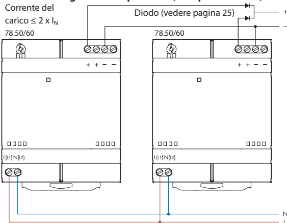
Collegamento in parallelo (solo per 78.50/60)
