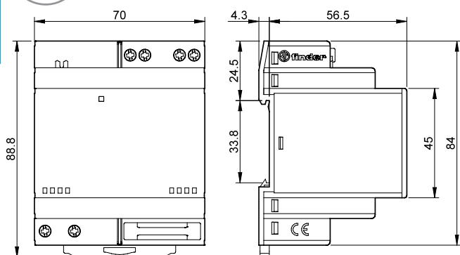
Tipo 78.1B Morsetti a vite
