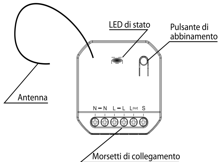
Il vostro Dimmer Smart Wi-Fi 9328
