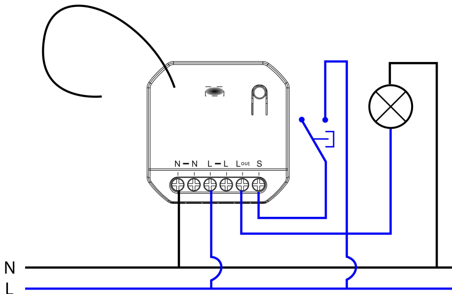
Lo schema di collegamento del 9328
