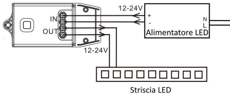
Lo schema di collegamento del 9330 con una striscia LED
