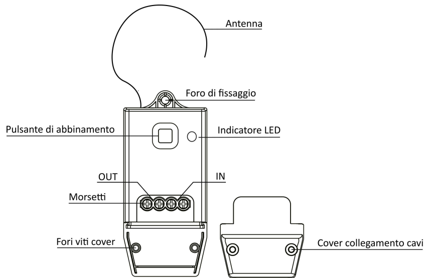
Il vostro Dimmer Smart Wi-Fi per strisce LED 9330
