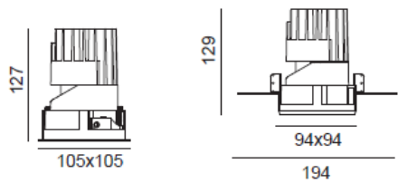
M1SF/C/./.../.. Versione con cornice With frame version M1SF/T./.../.. Versione trimless Trimless version
