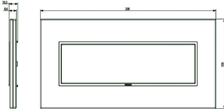
Vista ingombri
