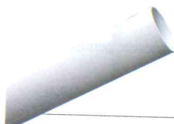
ACG8497 ASTA TONDA L=5,73m Ø100 mm spessore 2 mm NECESSITA DEL MOZZO ACG8539G L=6 m
