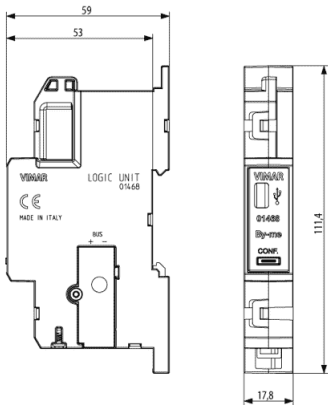
Vista ingombri
