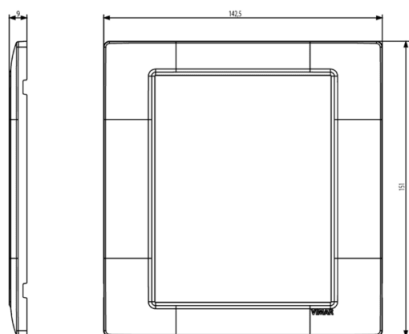
Vista ingombri
