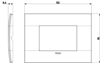
Vista ingombri
