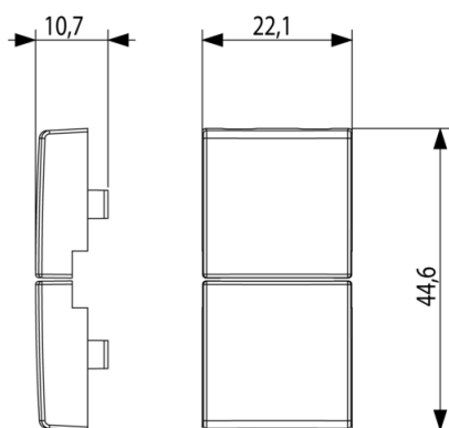
Vista ingombri
